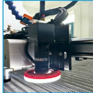
工业CCD相机 Industrial ccd camera
